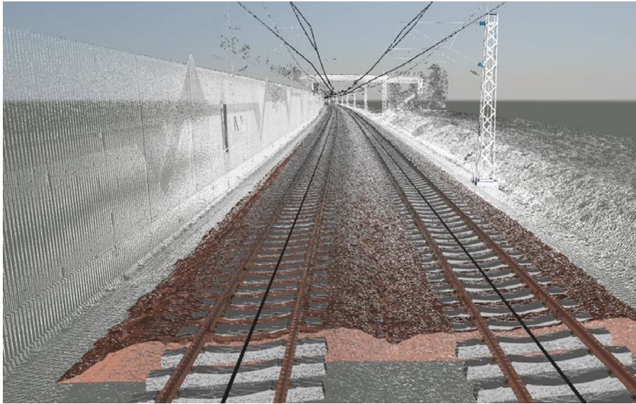
2: Bestandsmodell der SFS 4080
